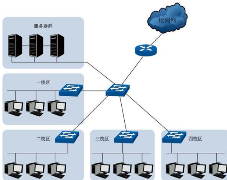
图 10-29 RIP 典型应用场景
