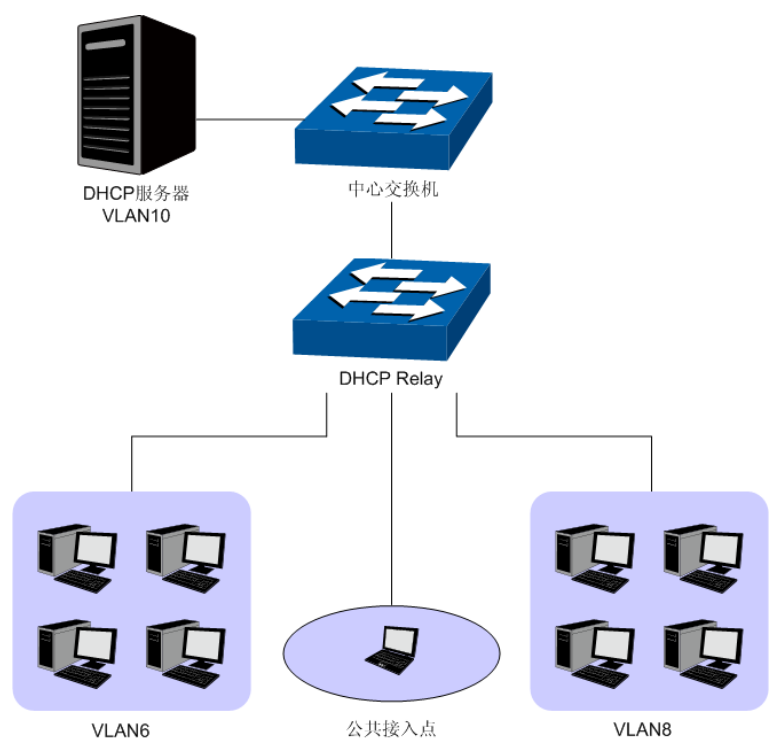
图 10-20 DHCP 中继典型拓扑图
