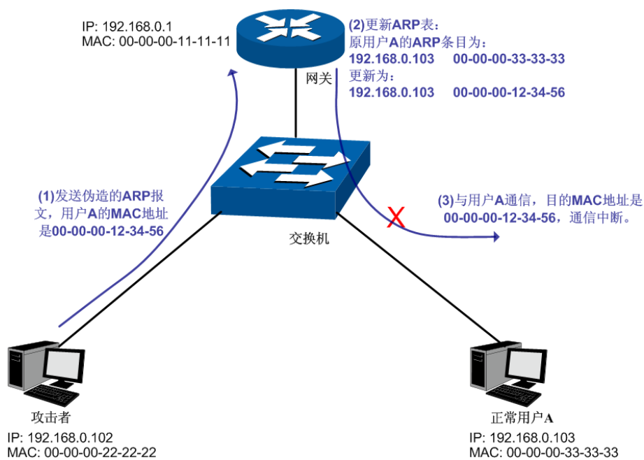
图 13-12 ARP 攻击-欺骗网关示意图
