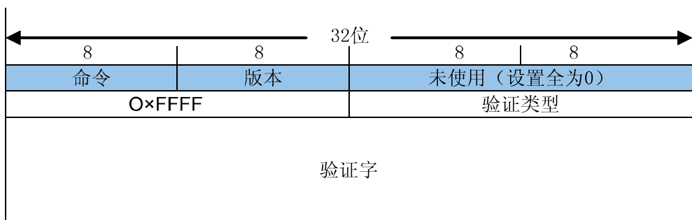
图 10-33 RIPv2 的认证报文格式
