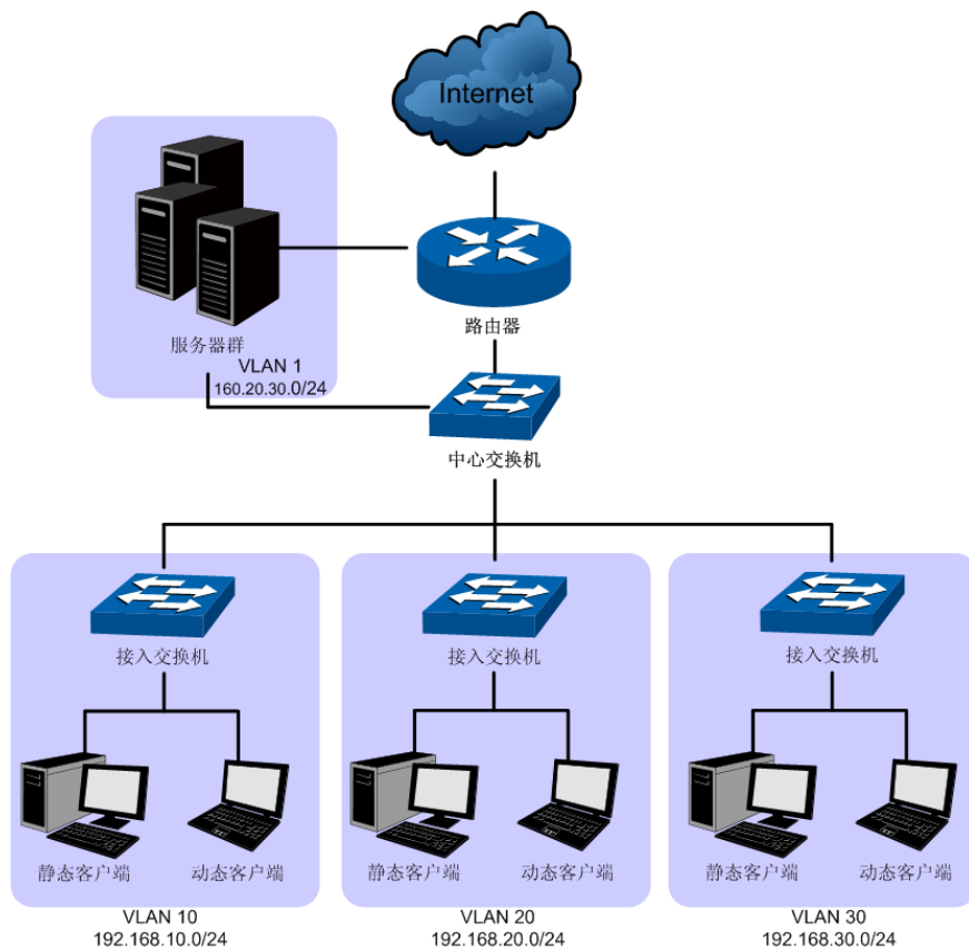
图 10-19 DHCP 服务器功能组网图
