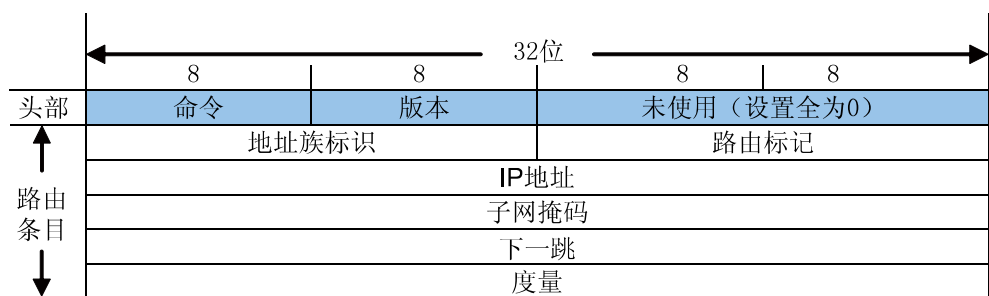
图 10-32 RIPV2 的报文格式
