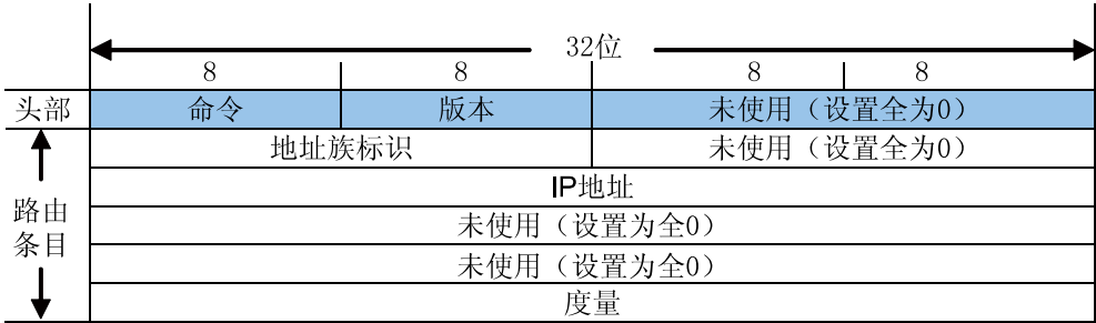
图 10-31 RIPv1 的报文格式
