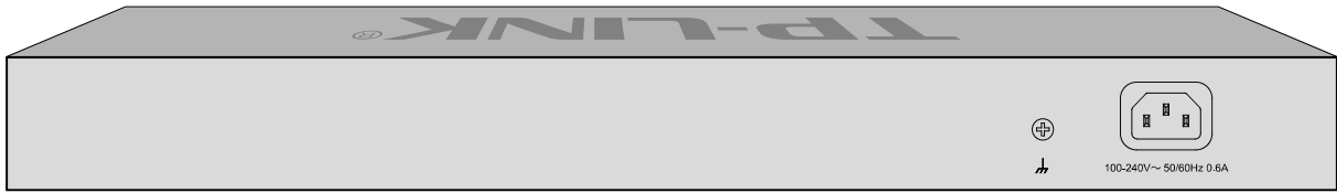
图 2-2 后面板
